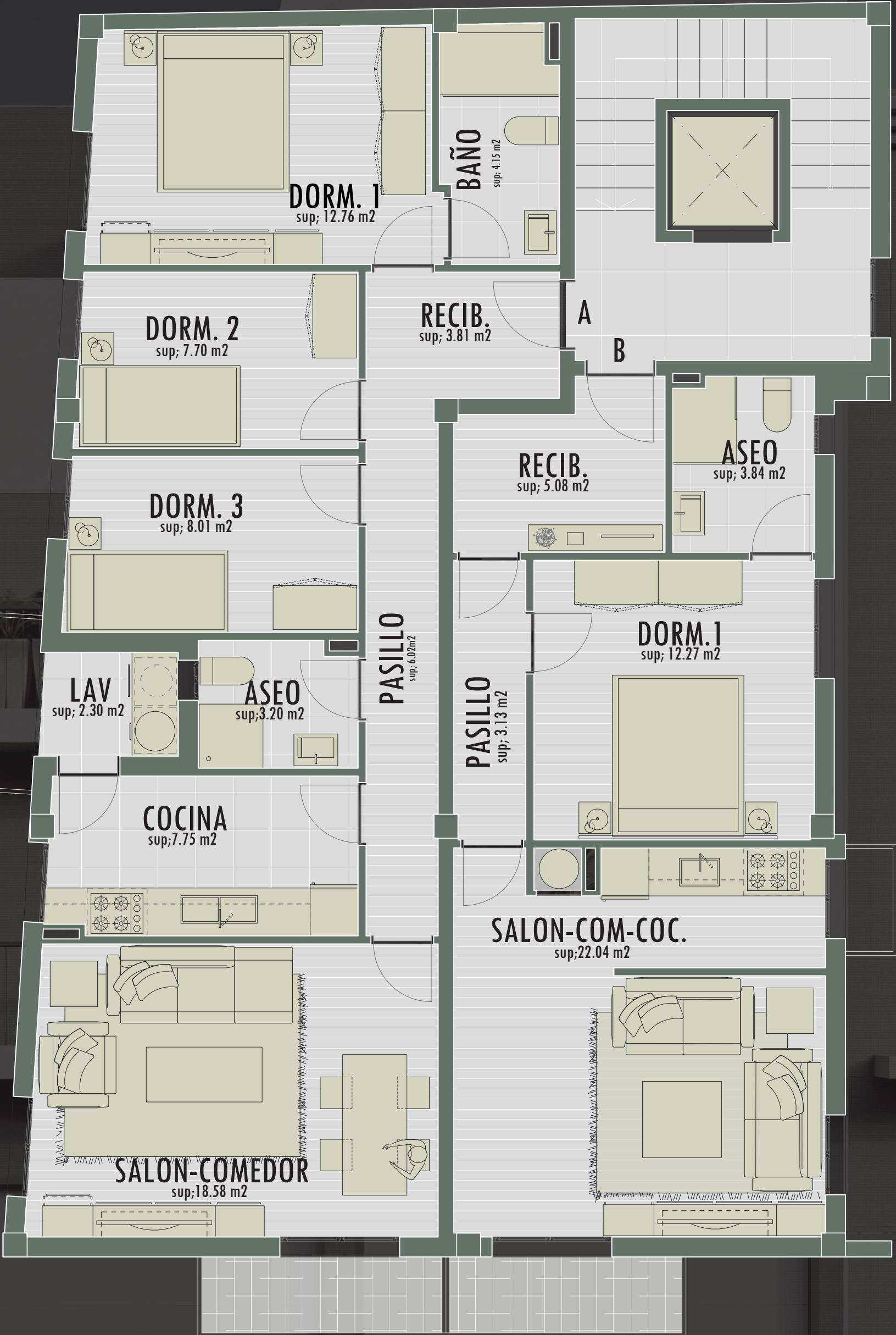
03. PLANTA SEGUNDA
